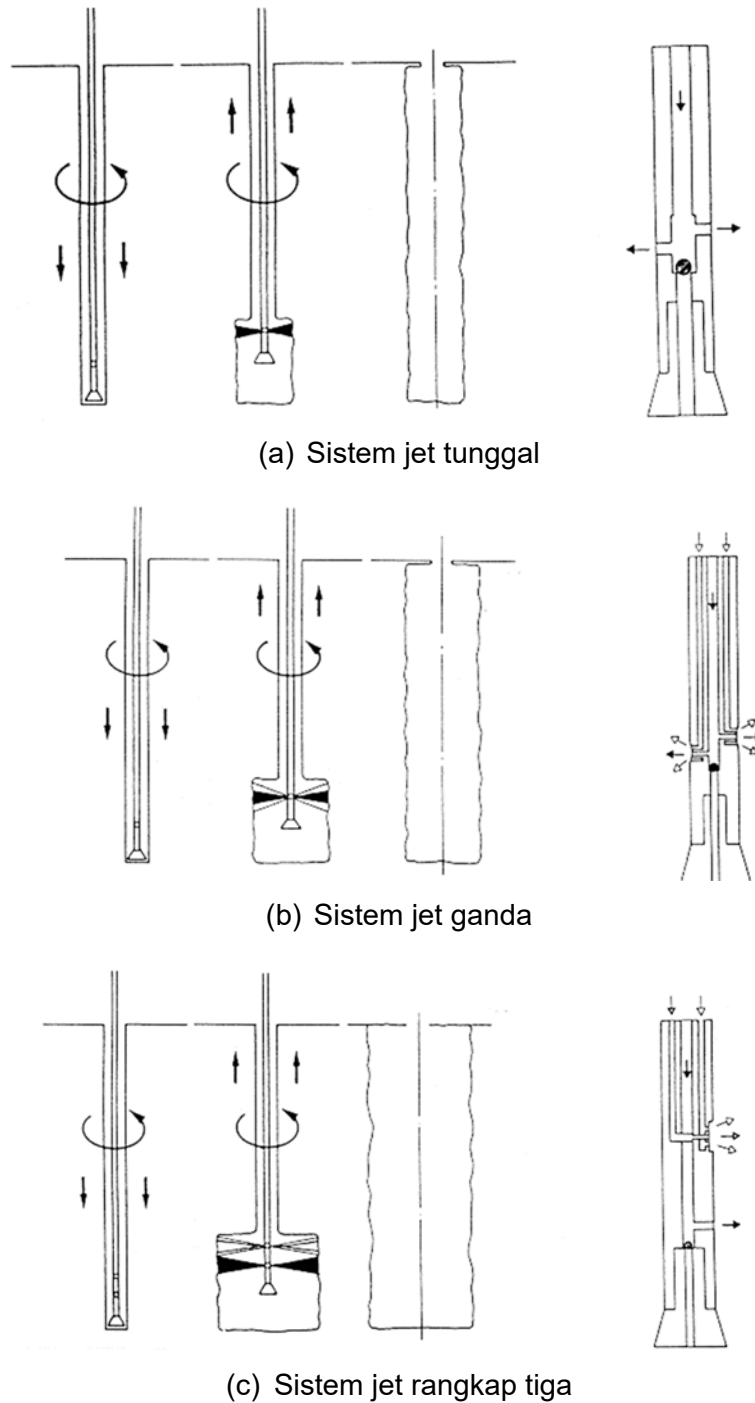
Gambar 4 - Sistem pengaliran jet grouting (BS EN 12716:2001)
