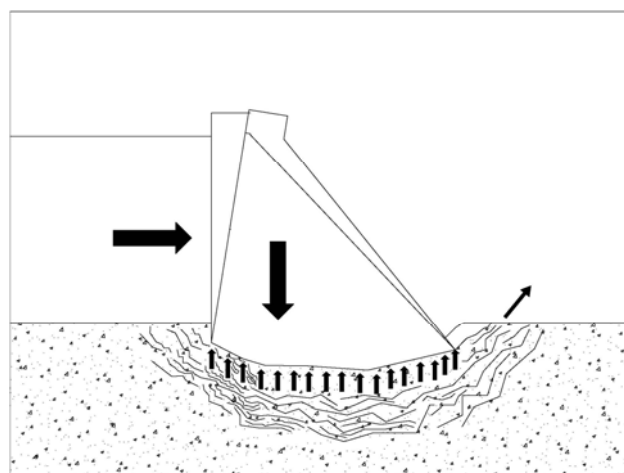
Gambar 75 – Keruntuhan pada fondasi bendungan beton oleh karena gaya apung
