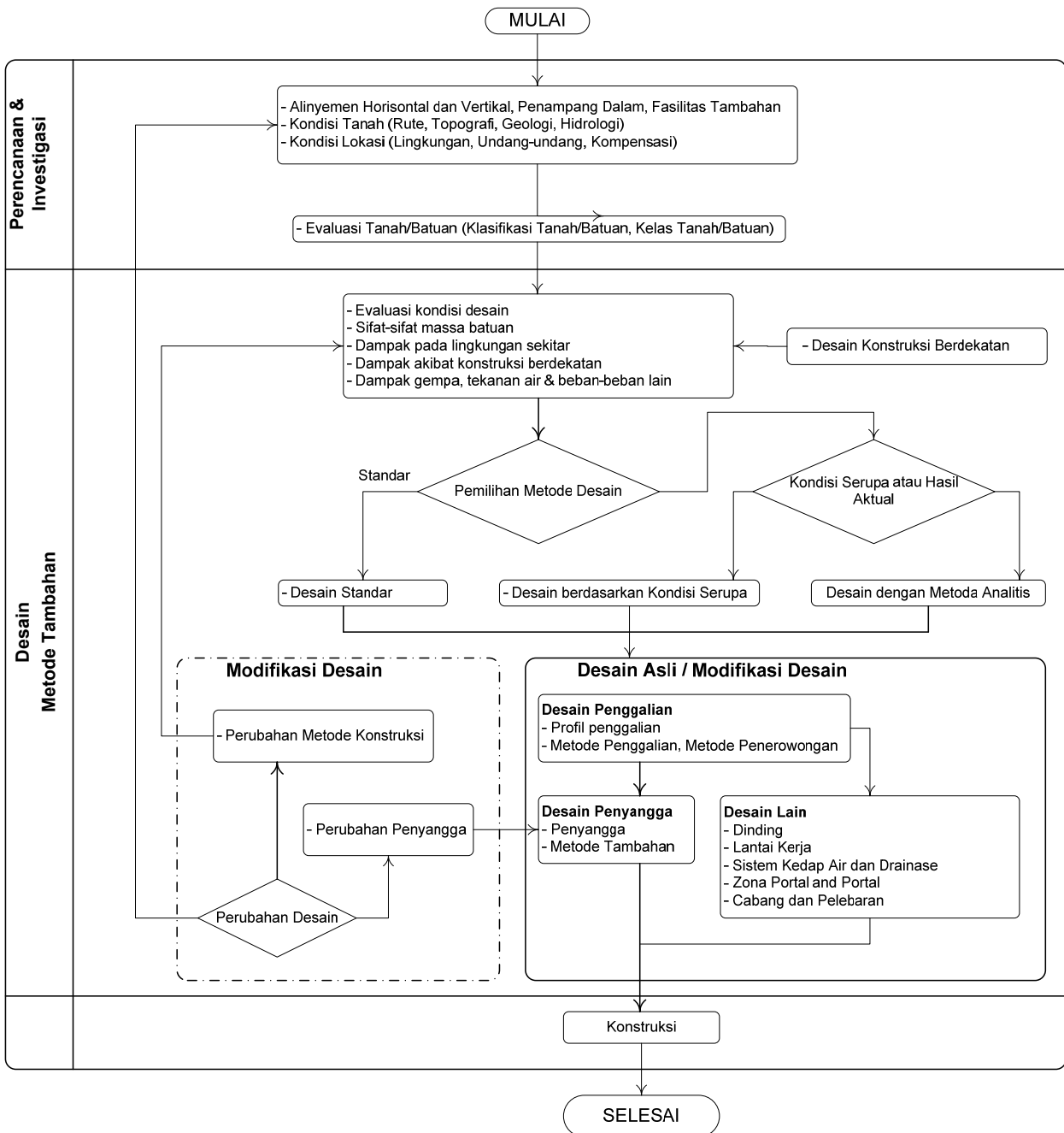
Gambar 19 - Prosedur perancangan terowongan pegunungan/batuan
