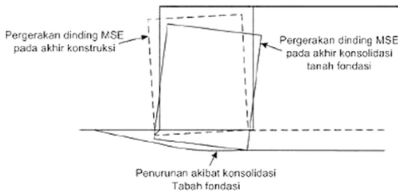
Gambar 58 – Pergerakan dinding MSE akibat penurunan konsolidasi tanah fondasi (GEO Hongkong, 2002)
